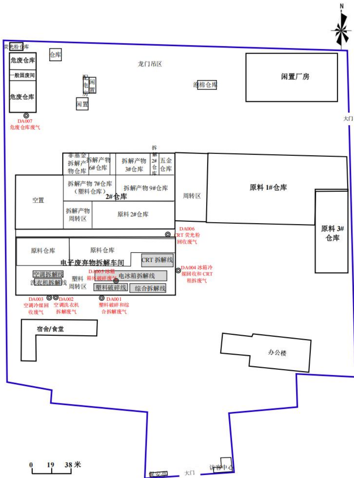
附图三 厂区平面布置图（改建前现有）
